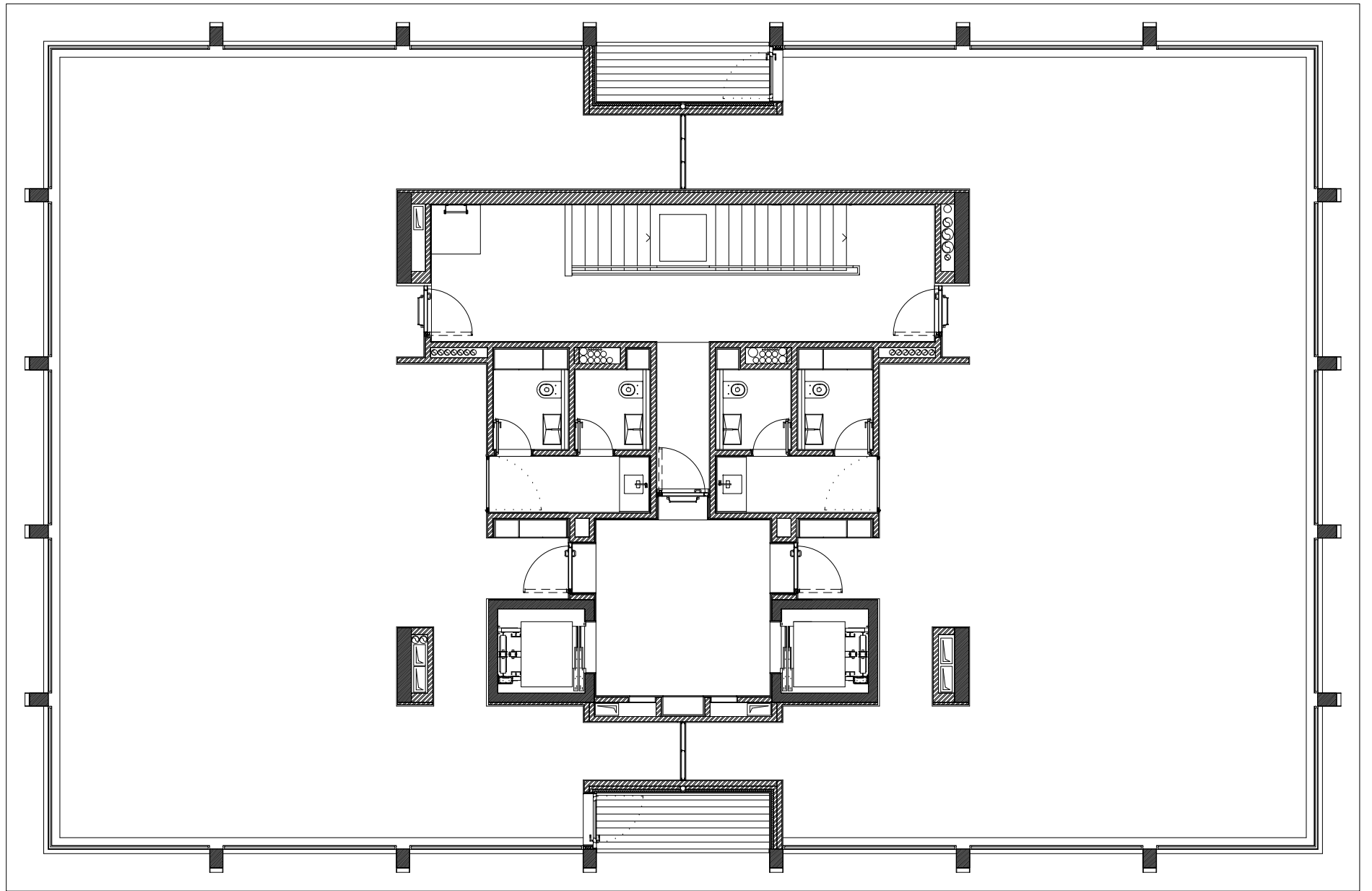
PLANTA PISO 6
