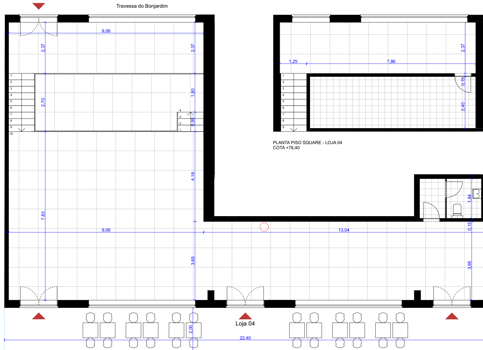
PLANTA PISO SQUARE - LOJA 04
