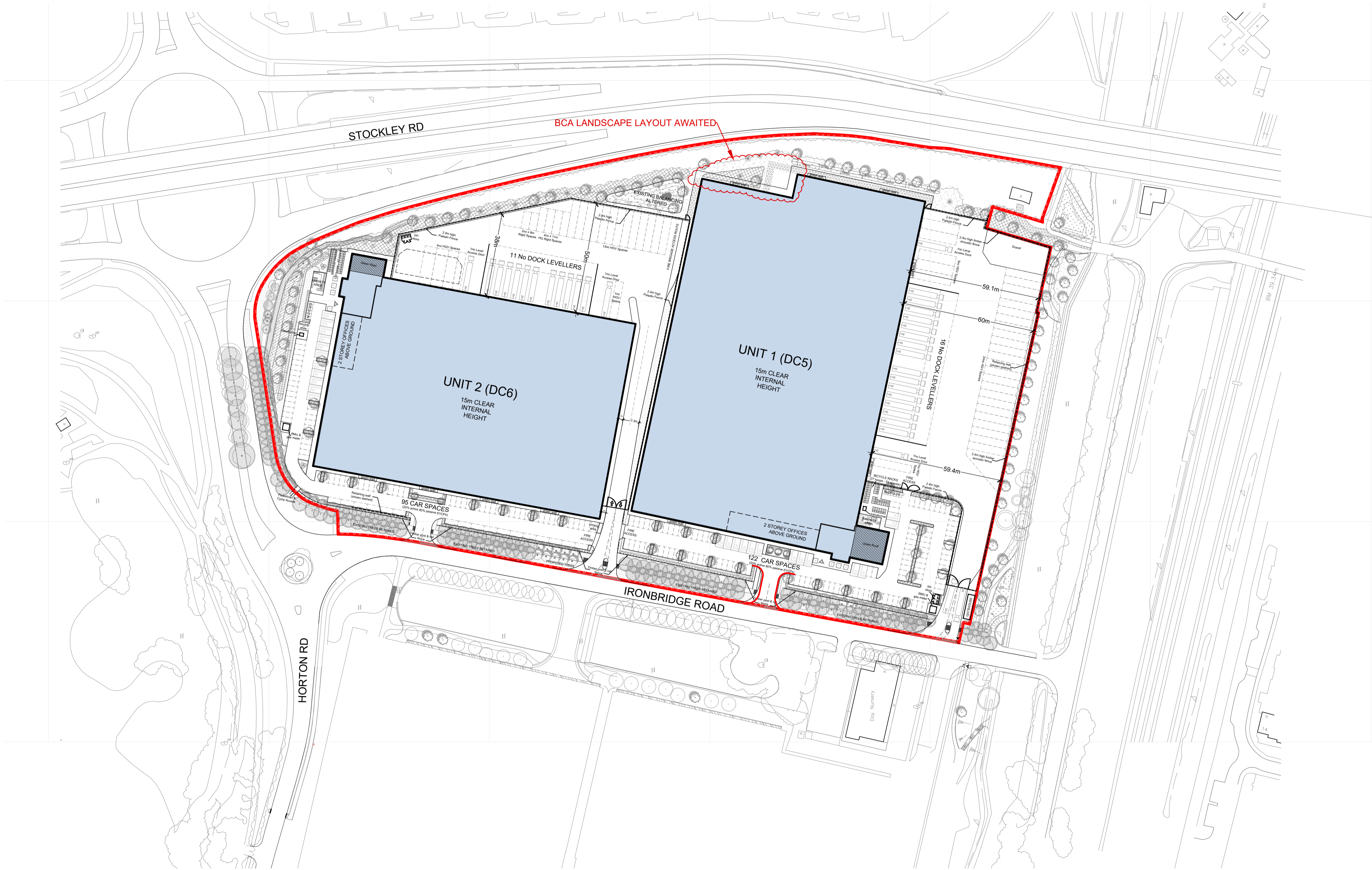
01 SITE LAYOUT 201 1:1000
